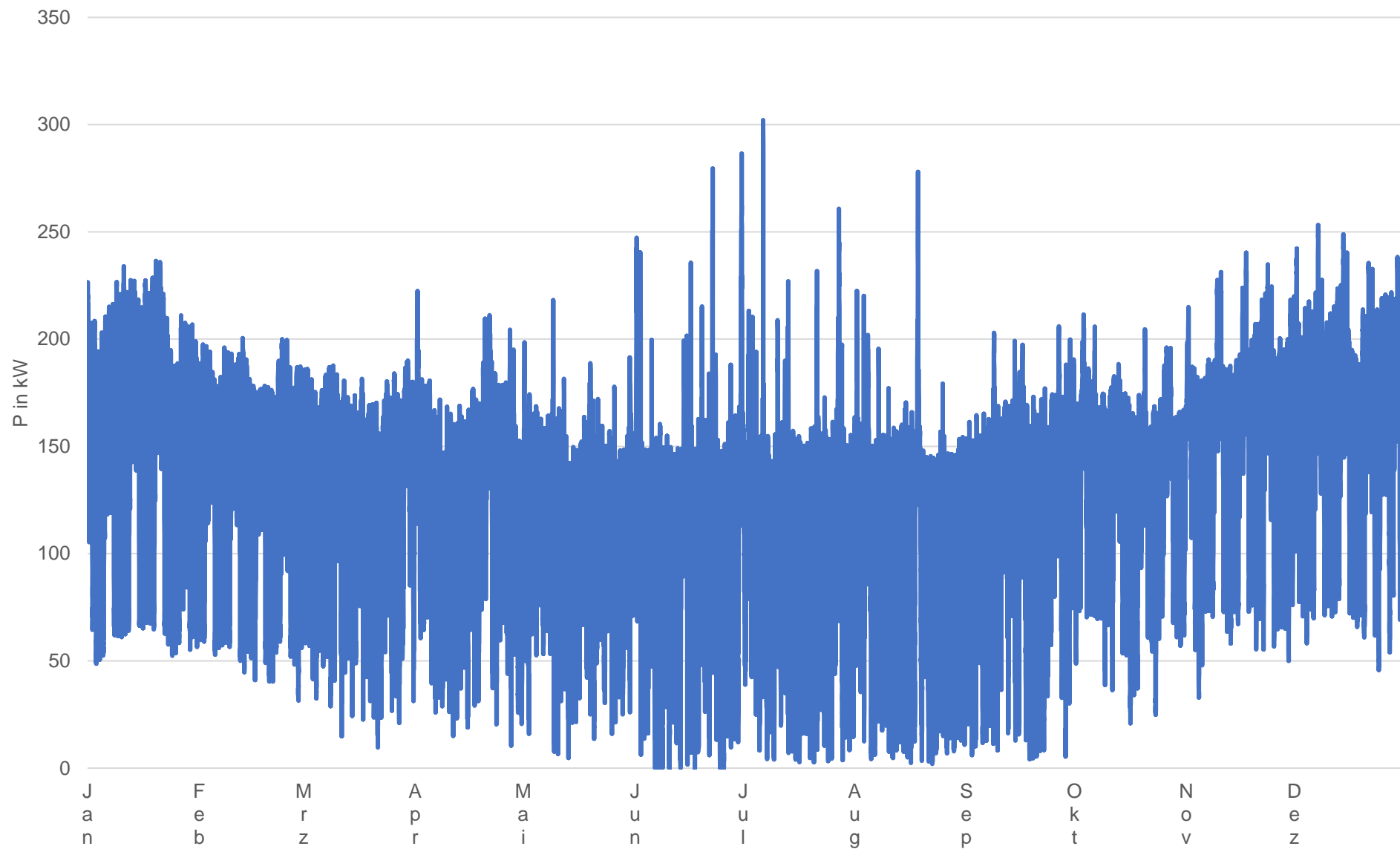
Summenlast der Netzverluste im Jahr 2024
